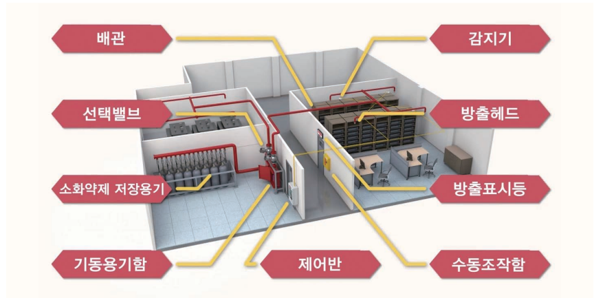
[그림 3] 이산화탄소 소화설비 구성요소
