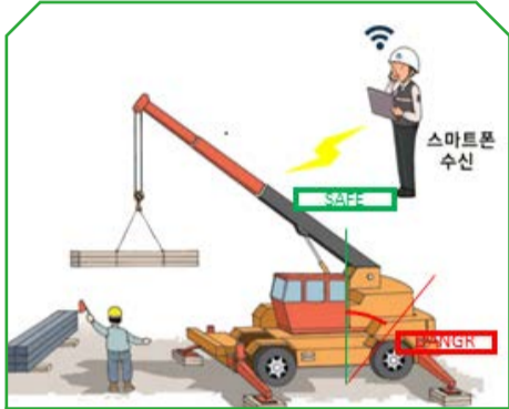
이동식 크레인 스마트 통합전도방지시스템
