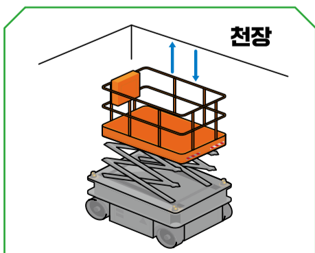
고소작업대 스마트 안전장치 (비접촉 과상승방지장치)
