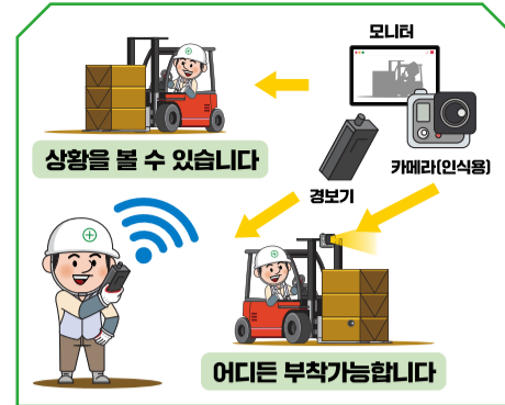
차량계 건설 및 하역운반기계 스마트 안전장치 (부착형 충돌방지)
